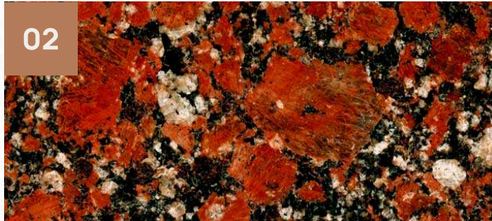
02 Капустинський граніт – Rosso Santiago с.12
