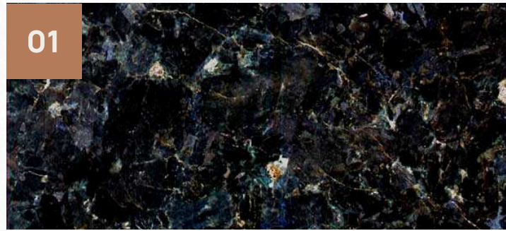
01 Лабрадорит – Irina Blue and Extra Blue Ukraine с.6
