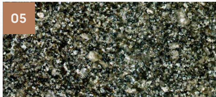
05 Старобабанський граніт – Pink Grey с.26
